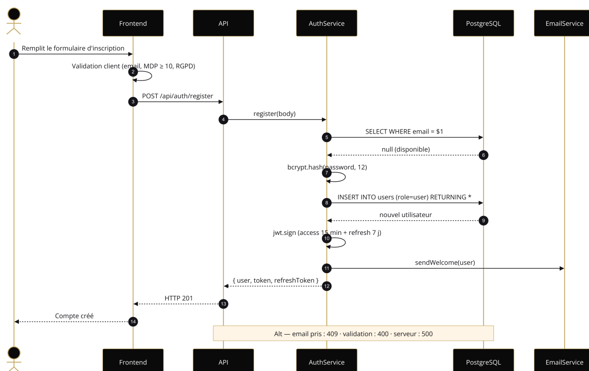
Figure 5 — Diagramme de séquence : inscription utilisateur
