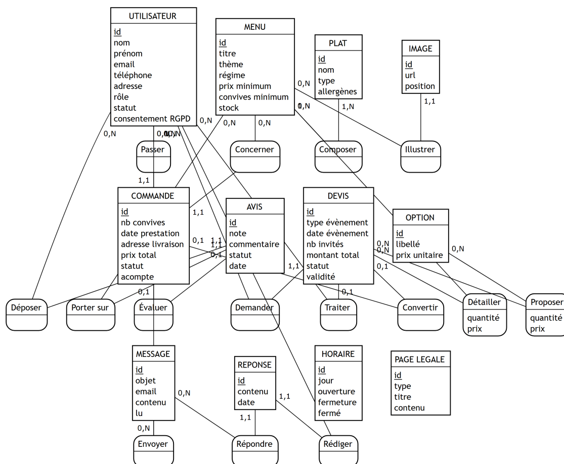
Figure 2 — Modèle Conceptuel de Données (MCD)
