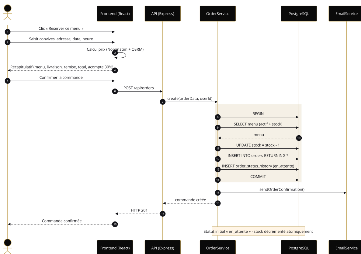
Figure 4 — Diagramme de séquence : commander un menu
